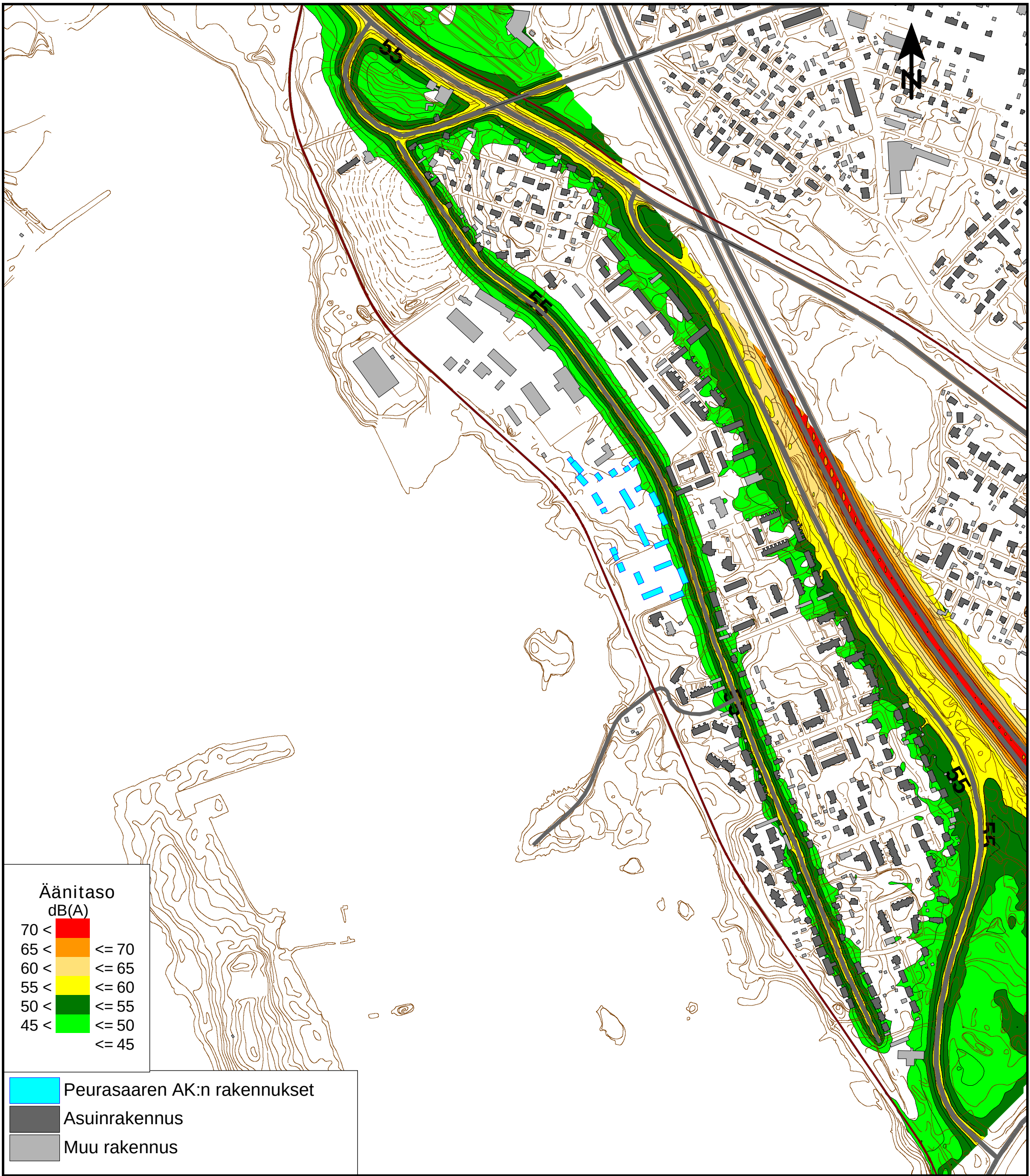
Kuva 8 Yöajan meluvyöhykkeet L_{Aeq\ 22-7}
