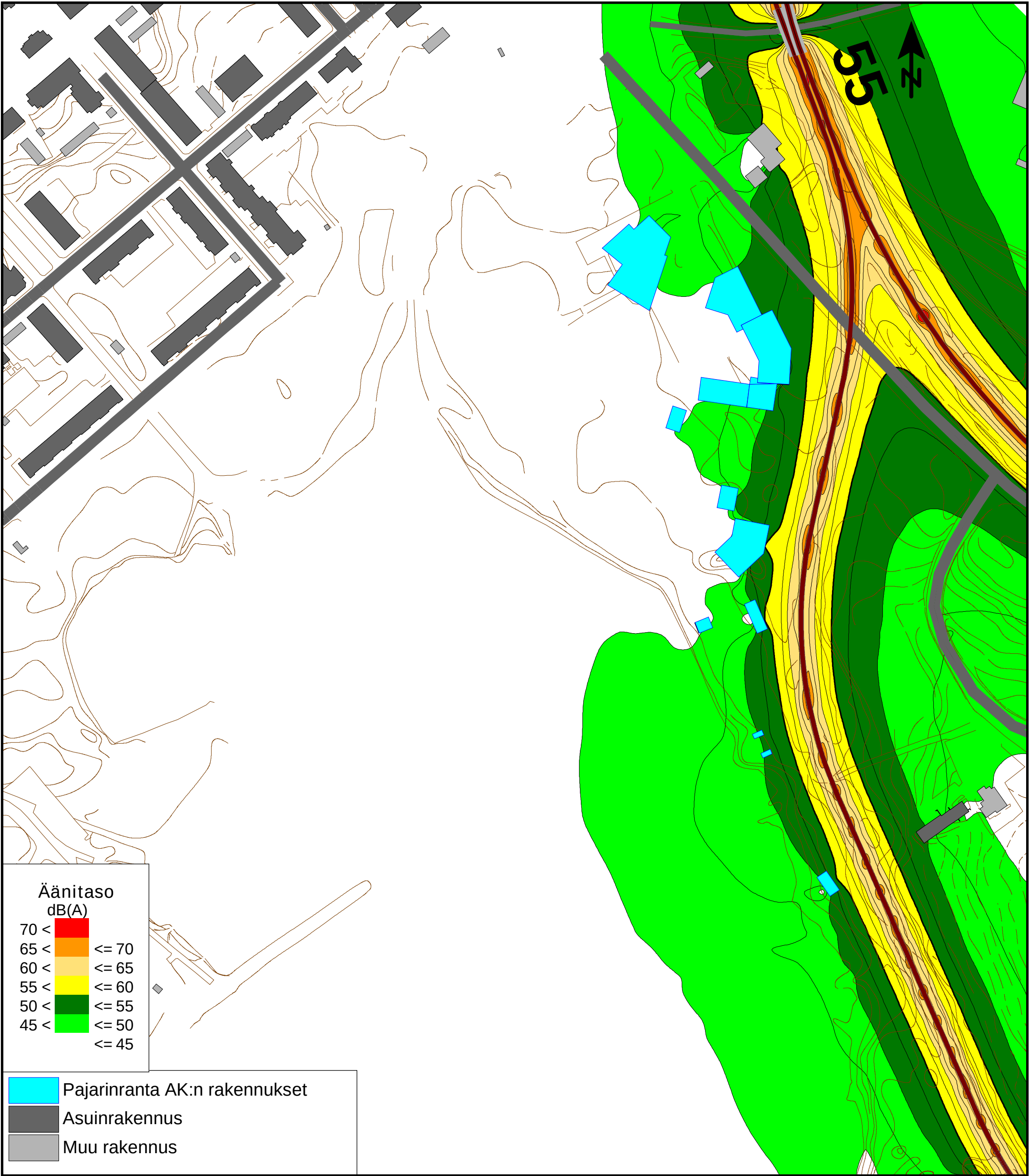
Kuva 17 Päiväajan meluvyöhykkeet L_{Aeq\ 7-22}
