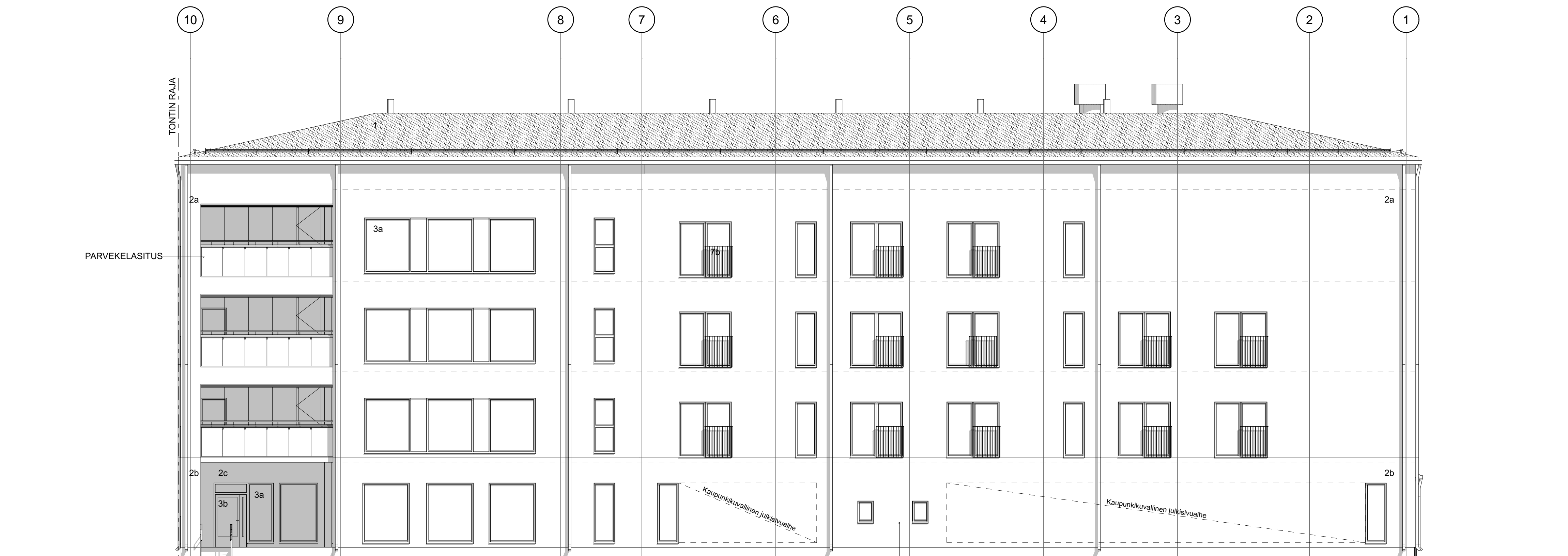
Julkisivu kaakkoon
